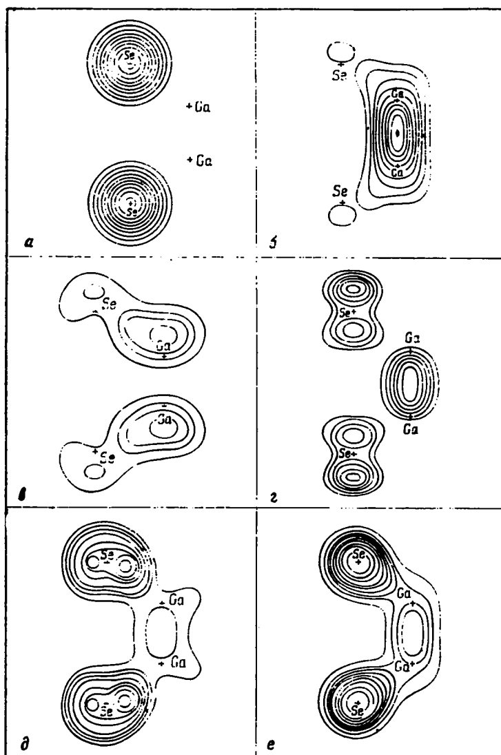
Рис. 6. Распределение электронов в пяти группах подзон в валентной зоне GaSe (a ÷ d) и распределение всех валентных электронов (e). [По Шлютеру (Nuovo Cim., 1973, v. 13B, p. 313).]
