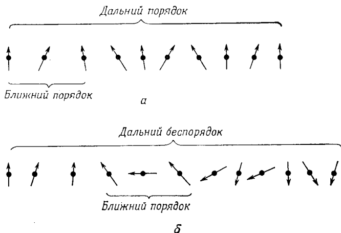
Фиг. 189. а — наличие дальнего порядка предопределяет наличие ближнего порядка; б — наличие ближнего порядка вовсе не означает, что имеется дальний порядок.
