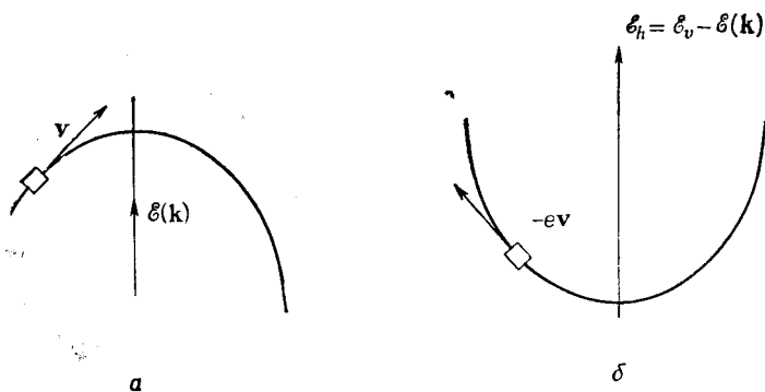
Фиг. 105. а — вакантное место в электронном распределении; б — соответствующая «дырка» (шкала энергии перевернута).
