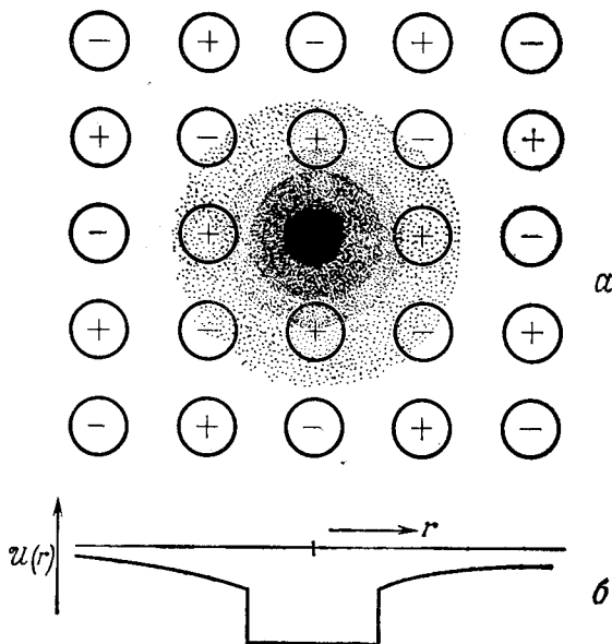
Фиг. 101. a — облако электронного заряда в F -центре; б — потенциальная яма в модели точечного иона.
