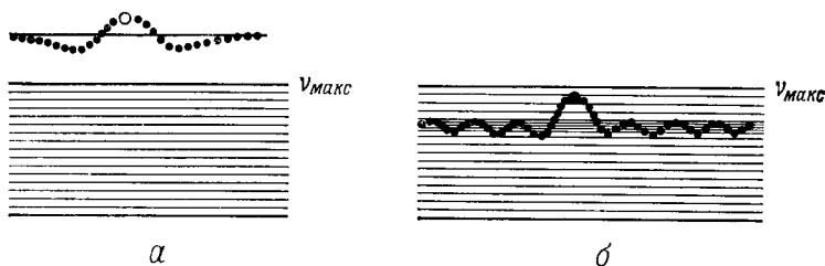
Фиг. 35. a — локальная мода колебаний легкой примеси, расположенная выше фоновой зоны; б — резонансная мода колебаний тяжелой примеси, расположенная внутри фоновой зоны.
