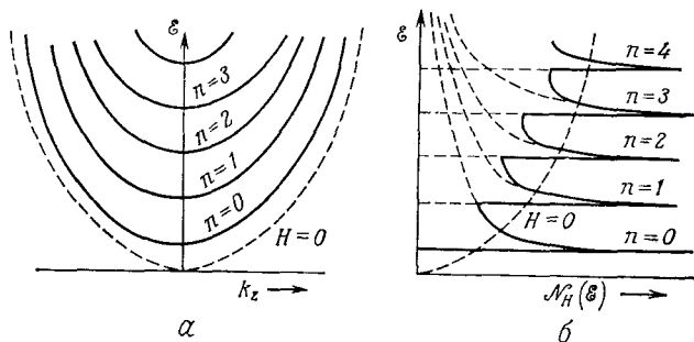
Фиг. 172. a — схема магнитного квантования для параболической зоны; б — плотность состояний.
