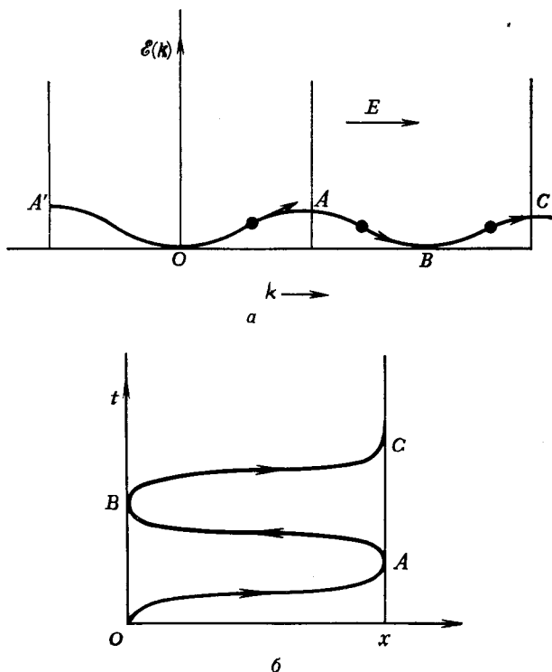
Фиг. 112. Электрон, движущийся в электрическом поле (одномерная модель).
