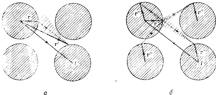
Фиг. 59. Обычная функция Грина (а), описывающая распространение волн из точки \mathbf{r}' в точку \mathbf{r} , заменяется структурной функцией Грина (б); последняя объединяет волны, идущие из всех эквивалентных точек решетки \mathbf{r}'' .
