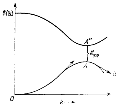
Фиг. 113. Вместо того чтобы идти к точке B , электрон может «перепрыгнуть» запрещенную зону и попасть в точку A'' .
