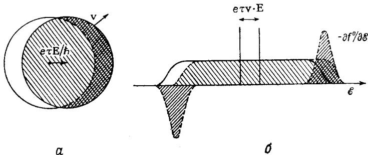
Фиг. 122. a — смещенная поверхность Ферми; б — смещенное распределение Ферми.
