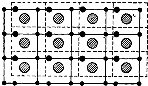
Фиг. 2. Различные возможности выбора элементарной ячейки.
