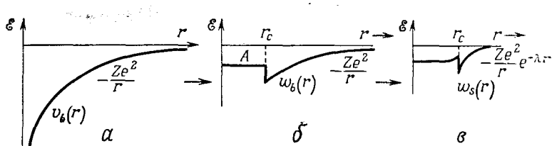
Фиг. 88. a — потенциал голого иона; b — псевдопотенциал голого иона; c — экранированный псевдопотенциал.
