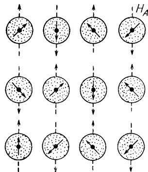
Фиг. 196. Оси квантования в антиферромагнитной системе.
