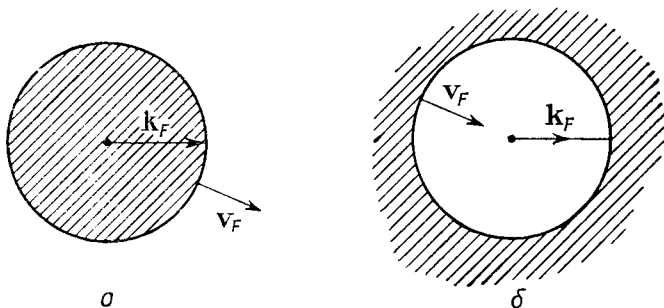
Фиг. 134. а — сфера «электронов» (масса m^* положительна); б — сфера «дырок» (масса m^* отрицательна).
