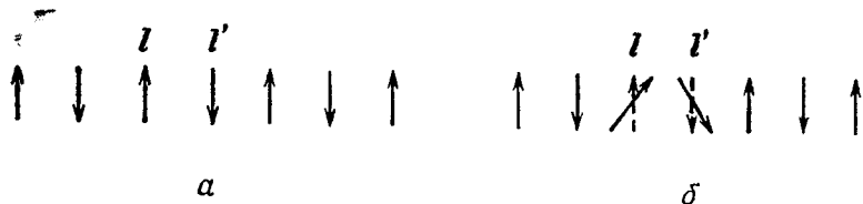
Фиг. 197. В антиферромагнитном упорядоченном состоянии (а) действие обменного оператора \mathbf{S}_l^\dagger \mathbf{S}_{l'} приводит к порождению двух спиновых отклонений (б).
