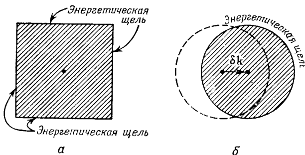
Фиг. 207. а — в полупроводнике энергетическая щель «привязана» к зоне Бриллюэна; б — в сверхпроводнике энергетическая щель переносится вместе с поверхностью Ферми.
