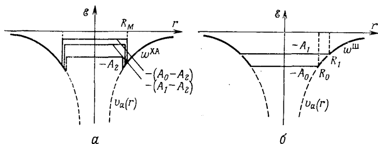
Фиг. 62. а — модельный псевдопотенциал Хейне — Абаренкова; б — модельный псевдопотенциал Шоу.
