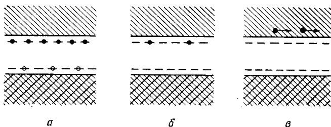
Фиг. 109. а — донорные и акцепторные уровни, занятые электронами и дырками; б — электроны и дырки рекомбинируют; в — избыточные электроны, термически возбужденные в зону проводимости.
