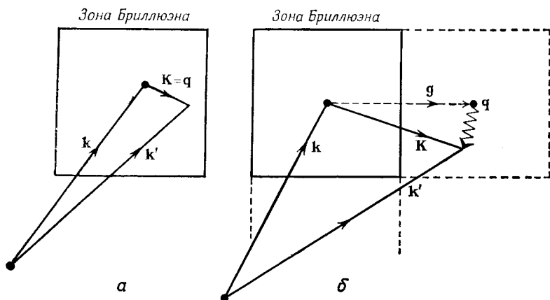
Фиг. 32. а — нормальные процессы; б — процессы переброса.
