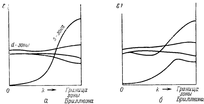
Фиг. 63. a — d -зоны, пересекающие s -зону; b — s — p -гибридизация.
