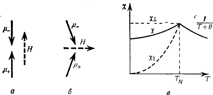
Фиг. 182. Магнитная восприимчивость антиферромагнетика.
