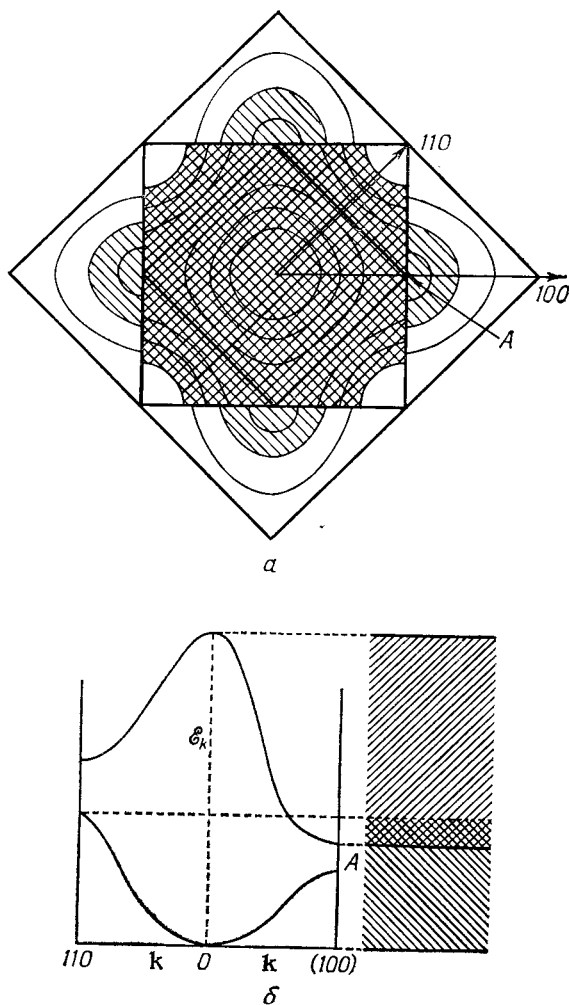
Фиг. 69. Перекрывание зон в двухвалентном металле.
