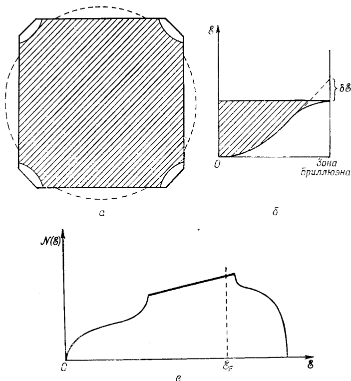
Фиг. 80. a — поверхность Ферми касается границы зоны; б — энергия понижается по сравнению со случаем свободных электронов; в — уровень Ферми проходит вблизи максимума плотности состояний.
