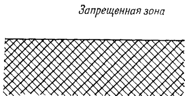
Фиг. 99. Примесные уровни.
