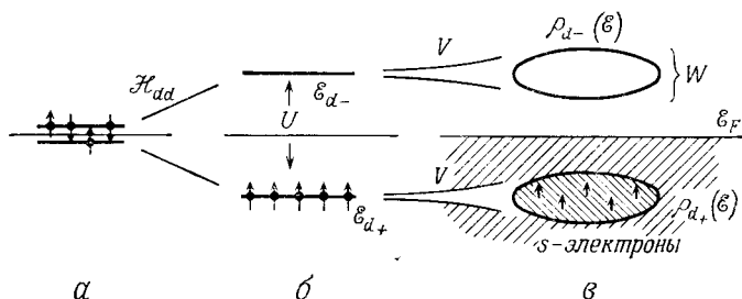
Фиг. 178. Атомные d -уровни (а) поляризуются и расщепляются из-за d-d -взаимодействия (б), а затем и уширяются, превращаясь в резонансные за счет гибридизации с s -электронами (в).
