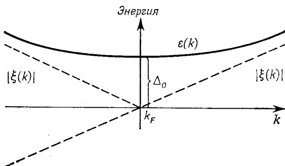
Фиг. 204. Энергия квазичастиц.
