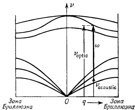
Фиг. 142. Многофононное поглощение.
