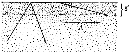
Фиг. 149. Эффективны только электроны, находящиеся в скин-слое.
