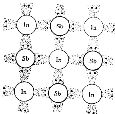
Фиг. 74. Антимонид индия (схематически).
