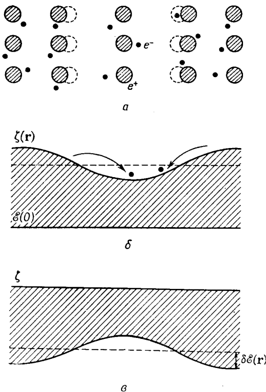
Фиг. 121. a — волны плотности в решетке приводят к изменению электронной плотности; б — уровень Ферми повышается или понижается; в — электроны перетекают таким образом, чтобы сохранить постоянным уровень Ферми; это приводит к возникновению деформационного потенциала.
