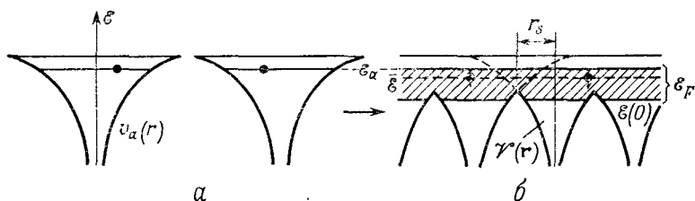
Фиг. 78. Модель Вигнера — Зейтца для расчета энергии связи.
