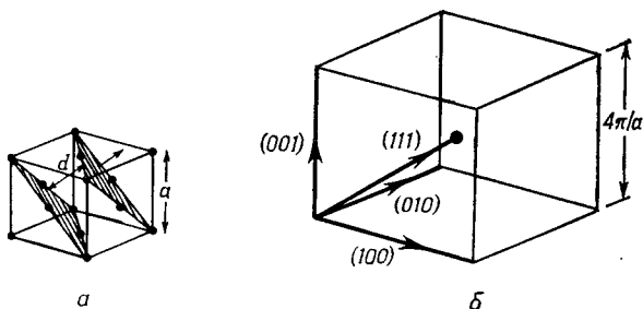
Фиг. 11. a — плоскости \{111\} в гранецентрированной решетке; б — соответствующая ячейка обратной решетки.
