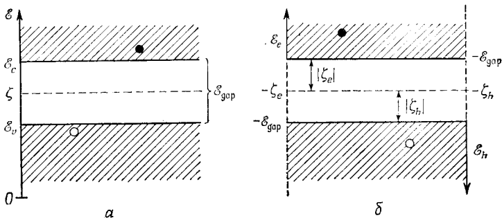
Фиг. 83. a — абсолютная энергетическая схема полупроводника; б — энергетические схемы для «электронов» и «дырок».
