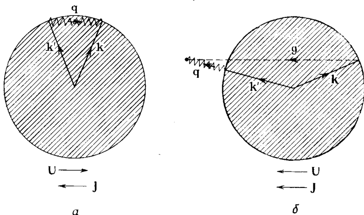
Фиг. 132. Увлечение фононов электронами. а — нормальные процессы; б — процессы переброса.
