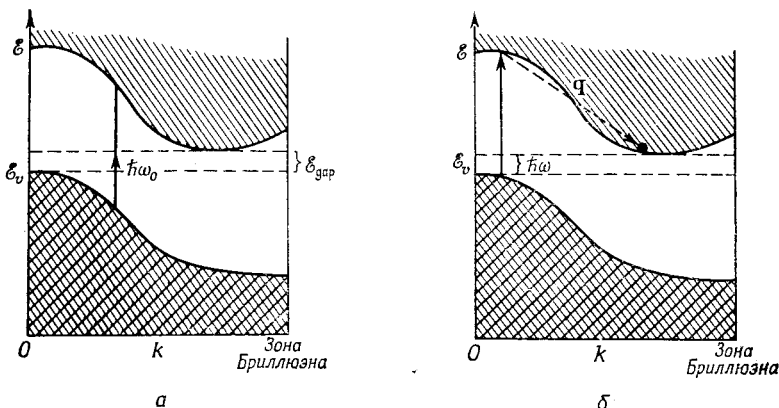
Фиг. 144. a — прямые переходы не обязательно соответствуют ширине запрещенной зоны; б — переход с участием фонона.
