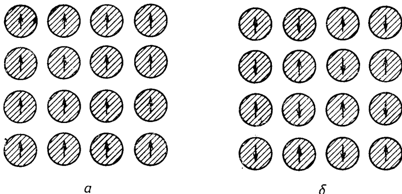
Фиг. 181. a — ферромагнитное упорядочение; b — антиферромагнитное упорядочение.
