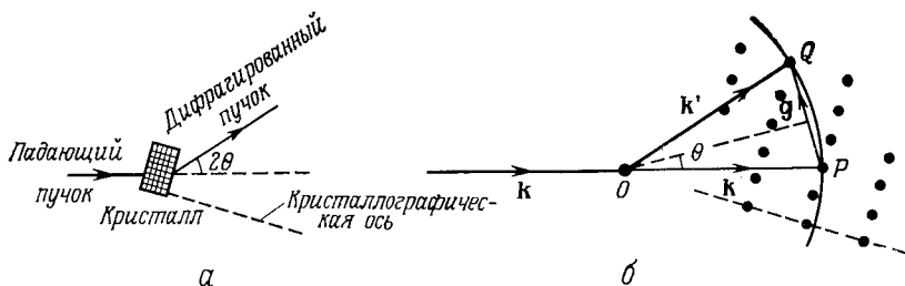
Фиг. 29. а — дифракция рентгеновских лучей; б — построение сферы Эвальда.
