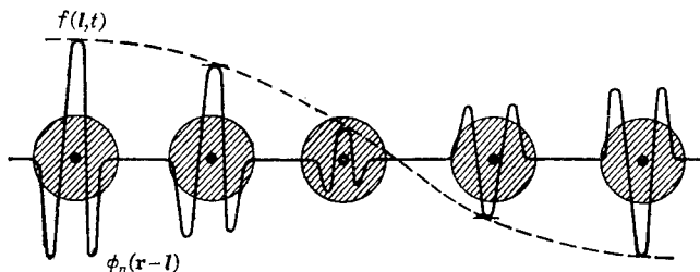
Фиг. 97. Волна, наложенная на атомные волновые функции.
