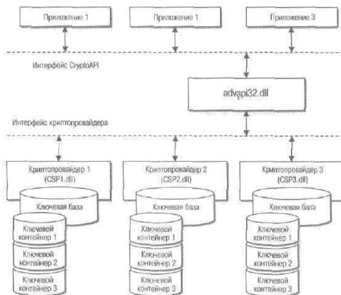
Рис. 2-1. Архитектура CryptoAPI 1.0
