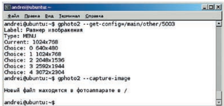
Рис. 2. Программа gphoto2 делает снимок.
