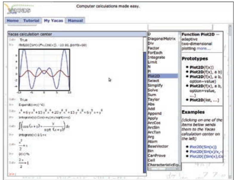
► Рис. 4. Web-интерфейс Yacas. Показан двумерный график и примеры некоторых аналитических преобразований.
