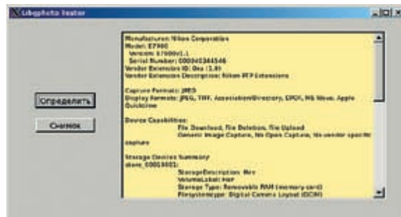
► Рис. 7. Программа libgphototester показывает возможности фотоаппарата Nikon Coolpix.
