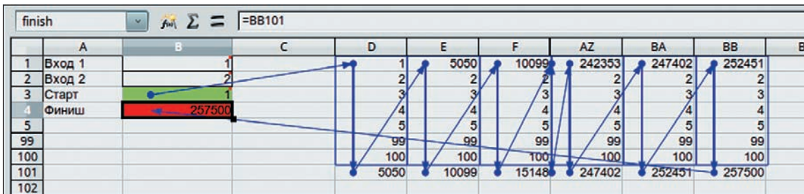
Рис. 2. Последовательность конвейеров SUM.
