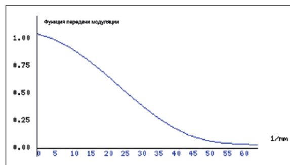
» Рис. 1. Функция передачи модуляции камеры на ПЗС.
